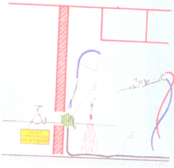
Rys.2. Spawane przewody, części maszyn i urządzeń oraz elementy konstrukcji budowlanych stykające się z materiałami palnymi lub przebiegające w pobliżu nich należy skutecznie chłodzić: 1-przewód doprowadzający wodę, 2-zwoje sznura z materiału niepalnego, 3-koc włókna szklanego.
