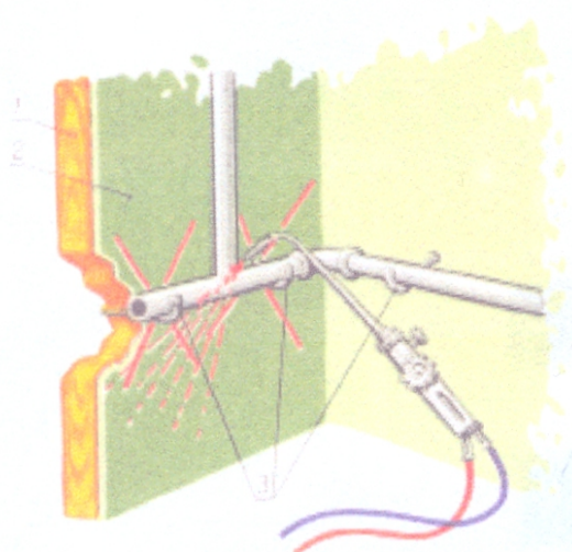
Rys.5. Elementy instalacji rozgrzewające się przy spawaniu od płomienia lub na skutek przewodnictwa ciepłego, stykające się z materiałami palnymi należy zdemontować lub skutecznie chłodzić: 1-palna ścianka, 2-niepalna wykładzina, 3-haki podtrzymujące instalację.
