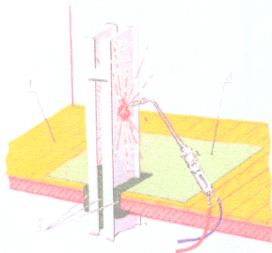
Rys.6. Sposób prawidłowego zabezpieczenia spawania metalowego elementu konstrukcji przechodzącego przez drewniany strop: 1-drewniany strop, 2-szczeliwo z materiału niepalnego, 3-koc z włókna szklanego.
